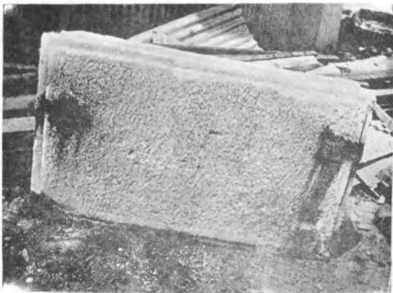
Εικών 7.—Δόμος κατηγορίας Β φέρων επί της τέως προσόψεώς του ύστερογενείς τετραπλεύρους συνδέσμους.
