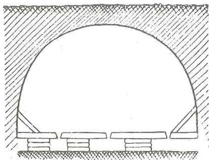
(Σχεδ. Γ). Τομὴ καὶ διάτρητον δάπεδον τῆς κρύπτης Ἁγ. Παντελεή- μονος Ἐνω Βοσπόρου.
